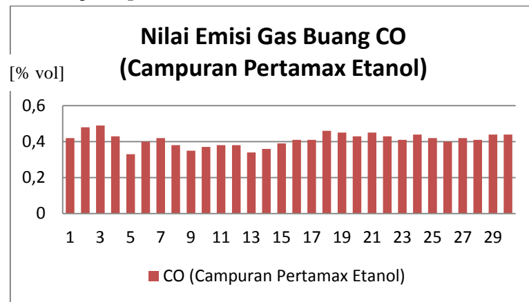
Gambar 5.2 : Nilai CO Bahan Bakar Campuran Pertamax Etanol
