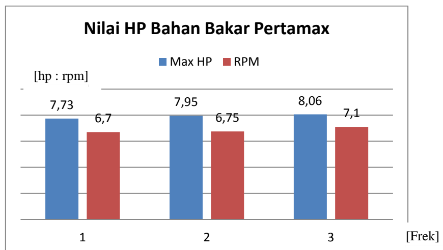
Gambar 5.9 : Nilai Horsepower Bahan Bakar Pertamina
