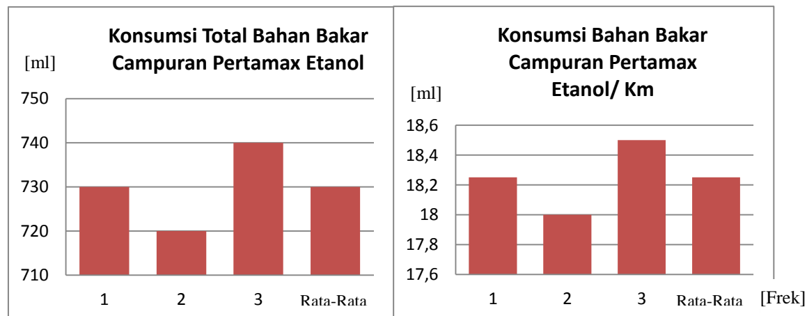
Gambar 5.7 : Konsumsi Bahan Campuran Pertamax Etanol
