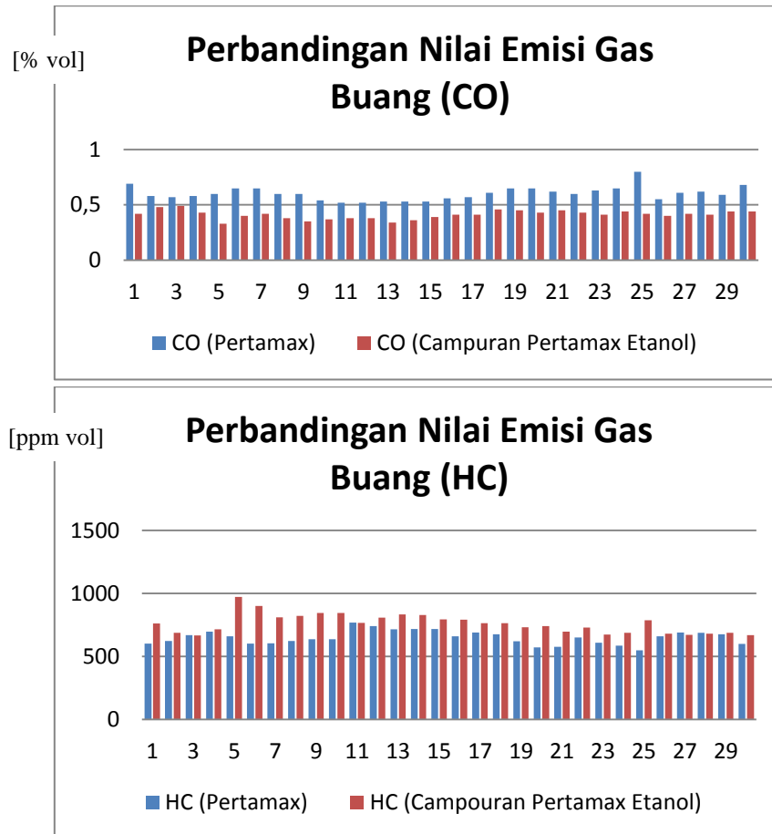
Gambar 5.5 : Perbandingan Nilai Emisi CO dan HC
