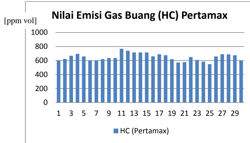
Gambar 5.3 : Nilai HC Bahan Bakar Pertamax
