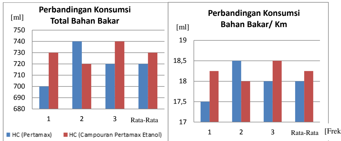
Gambar 5.8 : Perbandingan Konsumsi Bahan Bakar
