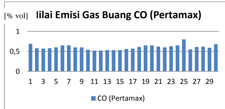
Gambar 5.1 : Nilai CO Bahan Bakar Pertamax
