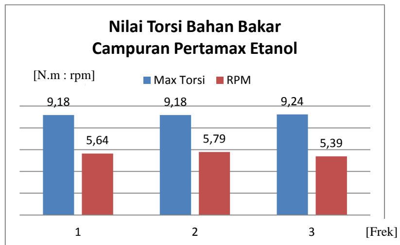
Gambar 5.12 : Nilai Torsi Bahan Bakar Campuran Pertamax Etanol
