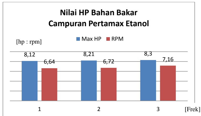
Gambar 5.10 : Nilai Horsepower Bahan Bakar Campuran Pertamax Etanol
