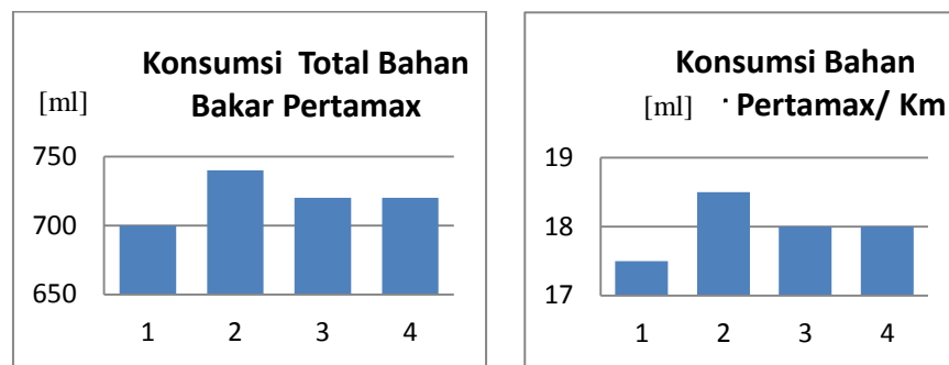
Gambar 5.6 : Konsumsi Bahan Pertamax
