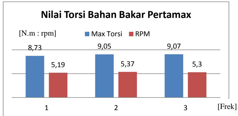
Gambar 5.11 : Nilai Torsi Bahan Bakar Pertamax
