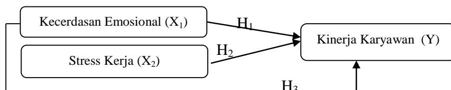
Gambar 1. Kerangka Konseptual
